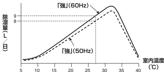
室内温度と除湿量の関係(湿度60%の時の例)
